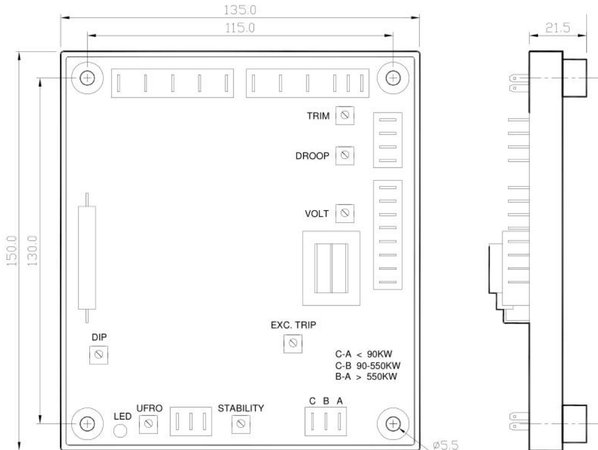
图一 尺寸图 UNITS:mm
